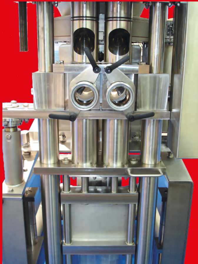
Ventile und Kolben ausgefahren für die Reinigung Product scrolls and valves run apart for cleaning
